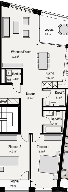
5b.12 3½-Zimmer-Wohnung NWF 101.7 m 2
